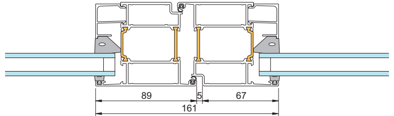
6 - Pardörrar, smalprofil
