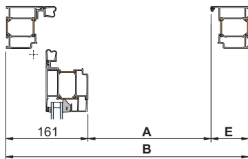
Dörr med klämfri bakkant
