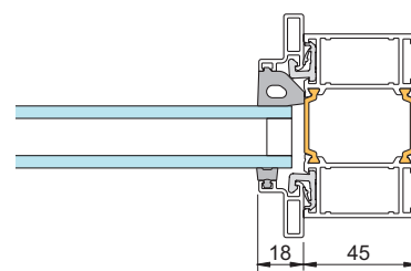
9 - Karmprofil
