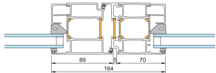
7 - Dörr med sidoljus. Smalprofil med bytbart anslag
