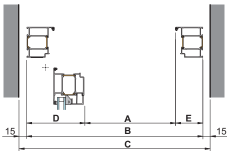
Anslagsgående dörr
