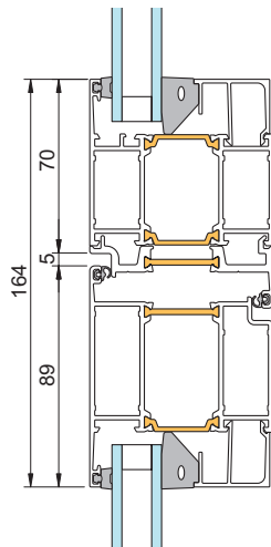
8 - Ö.K. dörr med överljus
