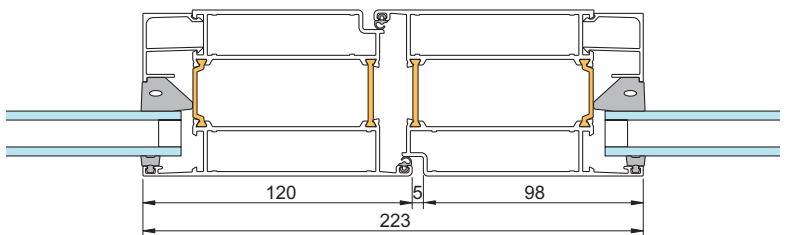
6 - Pardörrar, modulprofil
