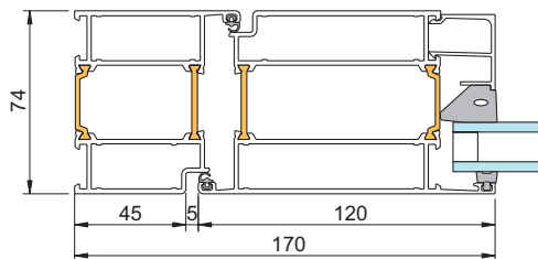
1, 2 - Dörr med modulprofil
