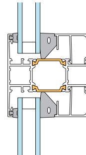
Glastjocklek 20-54 mm
