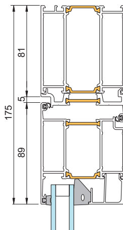
4 - Ö.K. dörr med profil för slagdörrsautomatik
