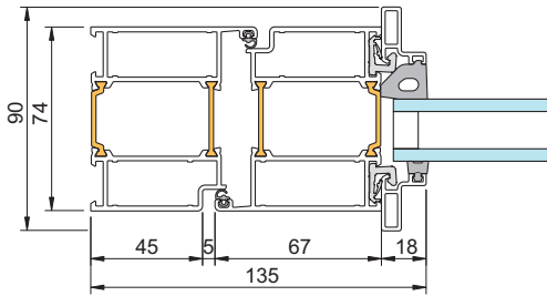
1 - Dörr med L-formad glasningslist.
