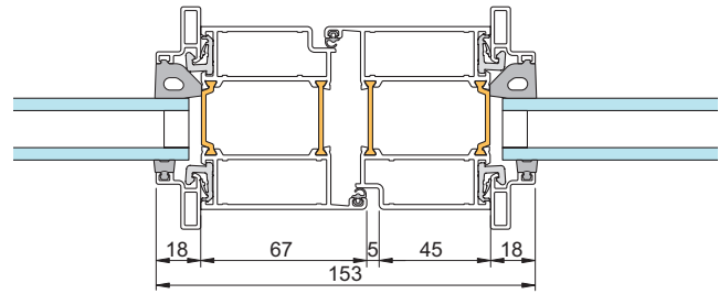
6 - Mötesdörrar
