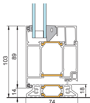
3 - Dörr med anslags-tätning mot fasad tröskel
