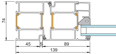
1, 2 - Dörr med smalprofil
