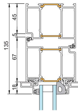
4 - Ö.K.dörr med karm
