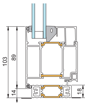
3 - Dörr med anslags-tätning mot tröskel
