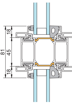
5 - Spröjs
