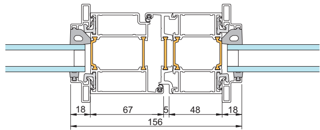
7 - Dörr med sidoljus
