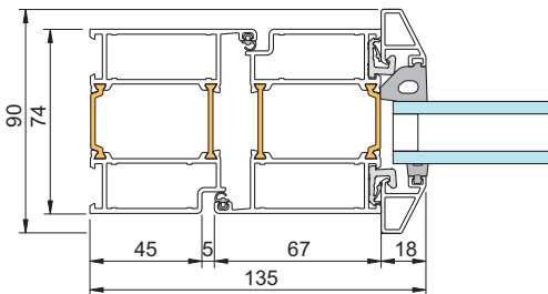
1 - Dörr med fasad glasningslist
