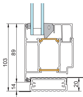
3 - Dörr med anslags-tätning mot rostfri isolerad tröskel
