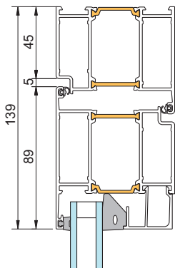
4 - Ö.K.dörr med karm
